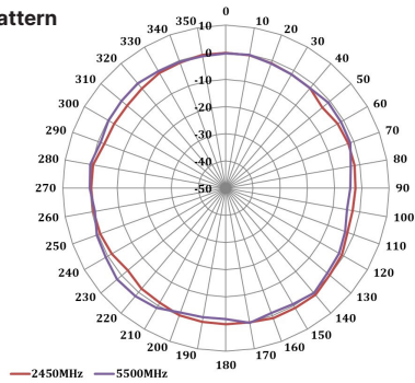
H-Plane Pattern
