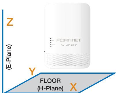
H-Plane Pattern
