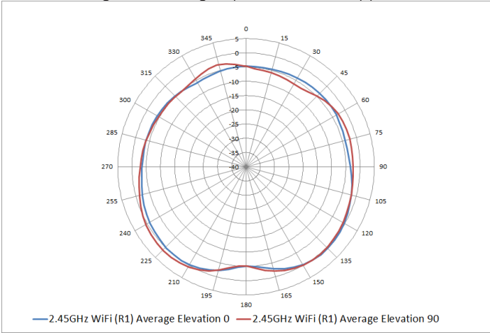
2.45GHz Wi-Fi (antennas 1, 2)
