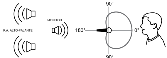
Locais Recomendados para Alto-Falantes para Microfones Cardiodes
