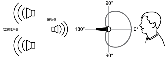
适用于心形话筒的扬声器推荐位置
