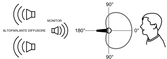
Posizioni consigliate degli altoparlanti per i microfoni cardiode
