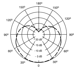
Corak Kutub Khas
