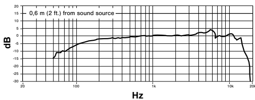
標準周波数特性
